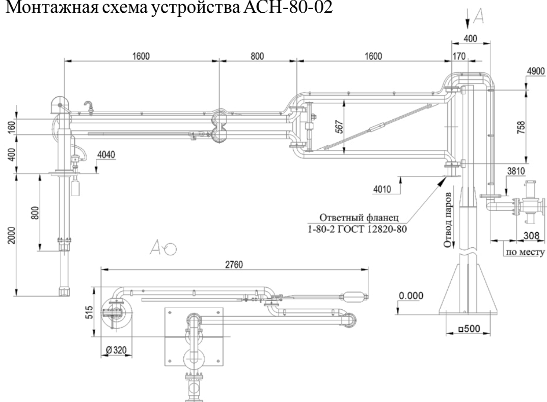
Монтажная схема устройства АСН-80-02
